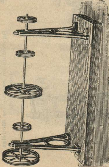
Transmission bâti fonte poulies nickel poli, sur planchette acajou verni.
