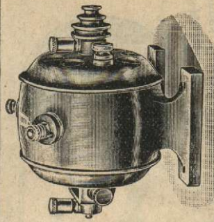
N° 260. Moteur Labor sur 110 volts alternatif ou continu. Corps et flasques aluminium poli, paliers anti-friction, graisseurs à godets, prises isolées, collecteur, force 1/60 HP. Constante garantie Dim. 120 × 90 × 80. Poids 900 gr. Prix 79 »
