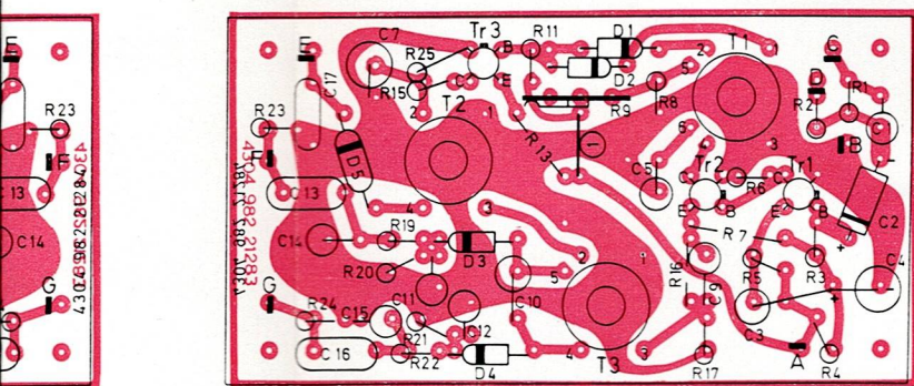
VUE CÔTÉ CUIVRÉ AANZICHT GEKOPERDE ZIJDE
