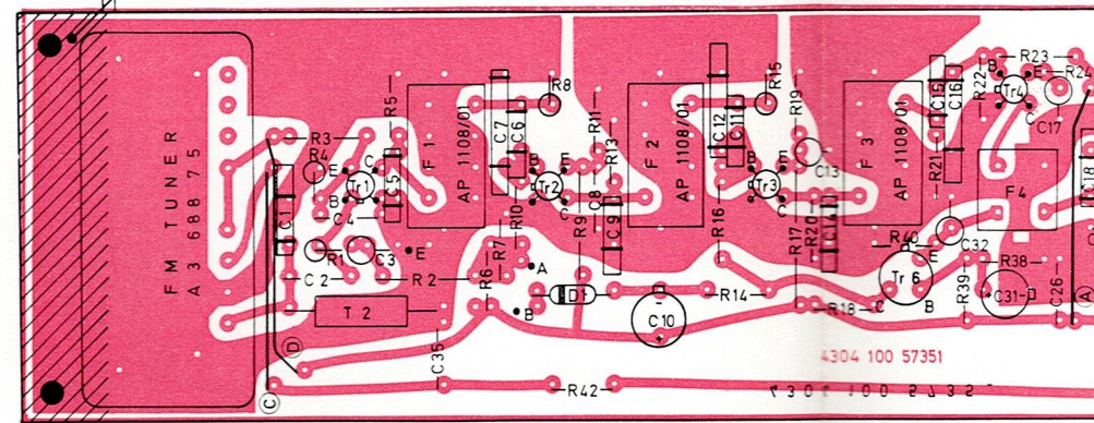
VUE COTE CUIVRE AANZICHT GEKOPERDE ZIJDE
