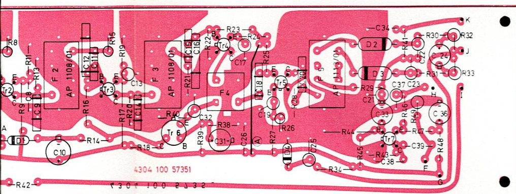
VUE COTE CUIVRÉ AANZICHT GEKOPERDE ZIJDE
