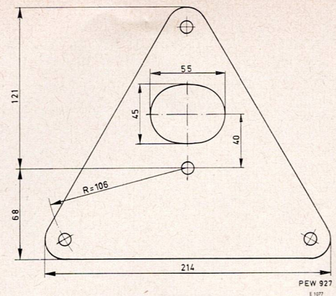
Fig. 3. Principal dimensions in mm Hauptabmessungen in mm Hoofdafmetingen in mm Dimensions principales en mm Dimensiones principales en mm
