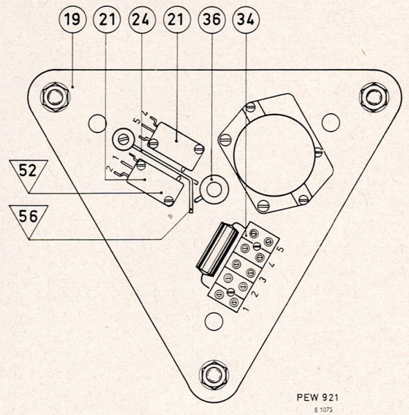
Fig. 2. Exploded view Zerlegtes Bild Exploded view Vue éclatée Vista en despiece
